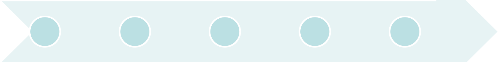
Medioevo Abaco
