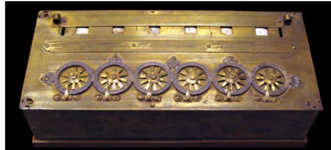
1642 Pascalina
