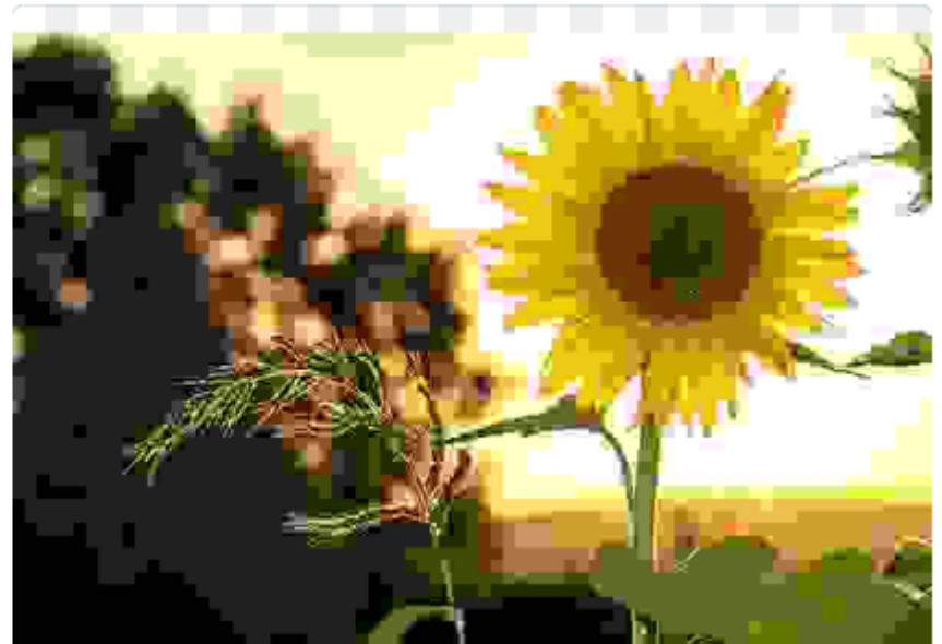
Qualità 0%
